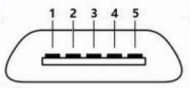
Micro USB 母头
