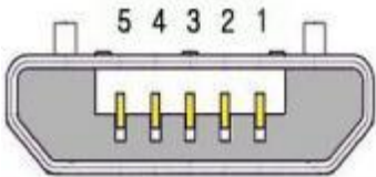
Micro USB 公头
